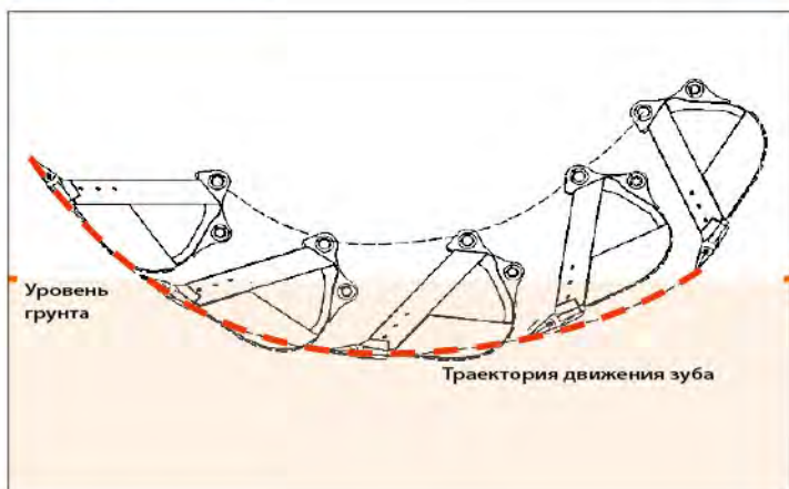
Стандартный ковш
